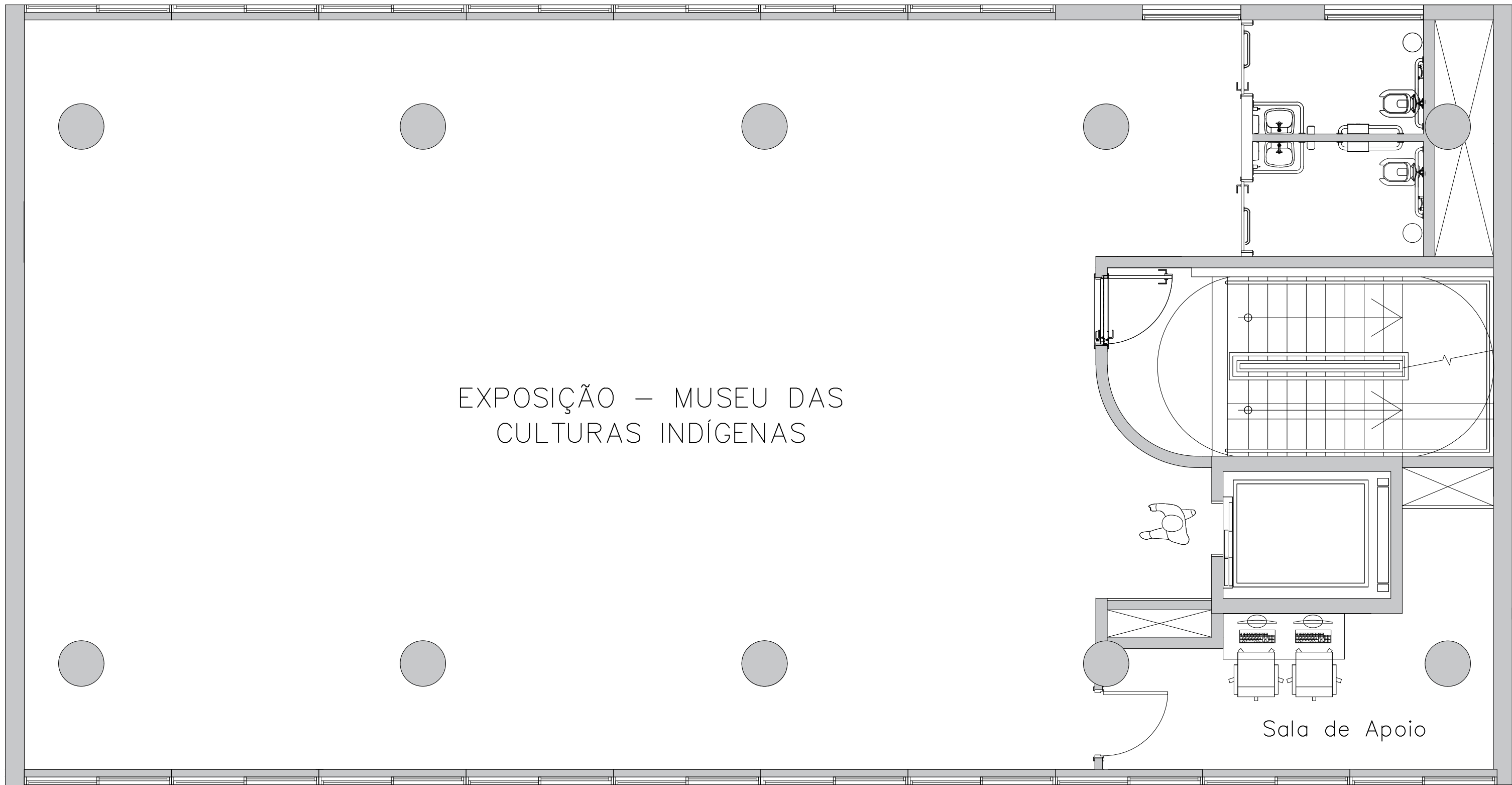
○ PLANTA BAIXA 4° PAVIMENTO
