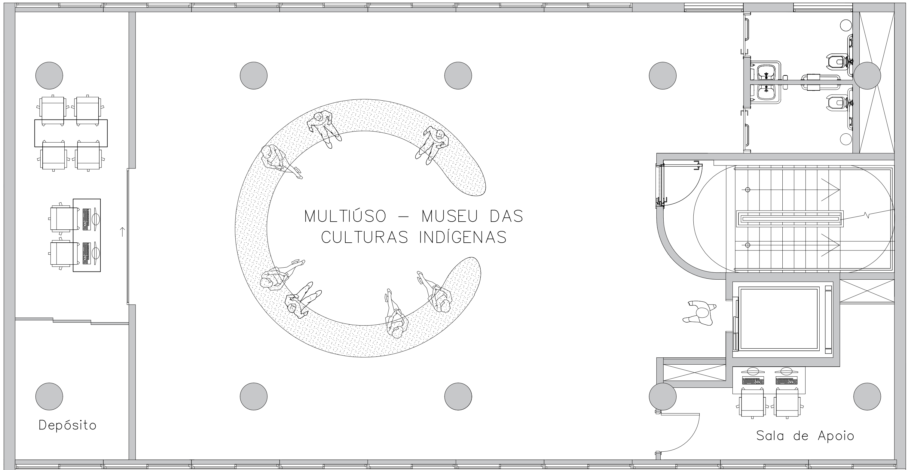
○ PLANTA BAIXA 7º PAVIMENTO
